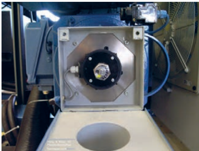
شکل ۱۸- تاکومتر
