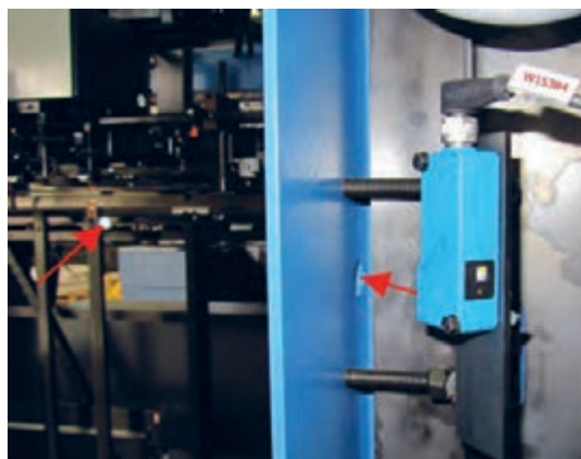
شکل ۲۲- حسگر نوری تشخیص محدوده کاغذ
