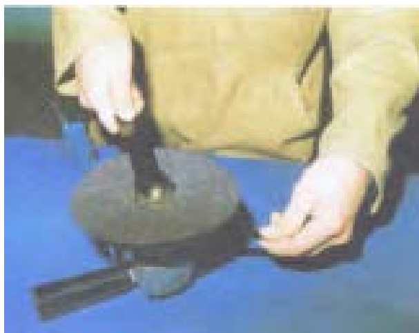
شکل ۷-۳۸- نمونه گرفتن آپارهای مخصوص به منظور باز یا بستن مهره صفحه.
