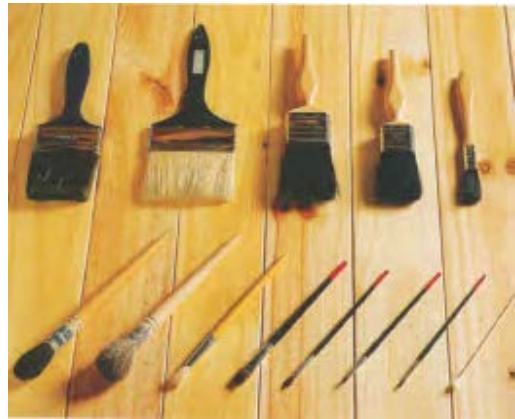
شکل ۴-۲۹- انواع قلم‌مو.
