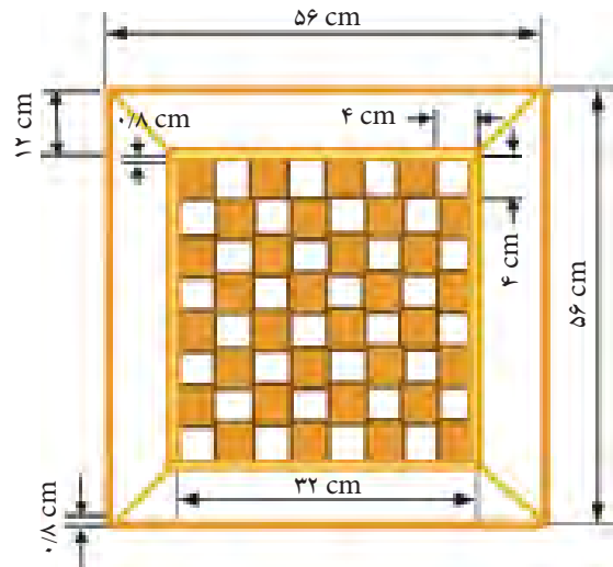
شکل ۱۵۹-۱۲. دو نمای اصلی میز شطرنج.
