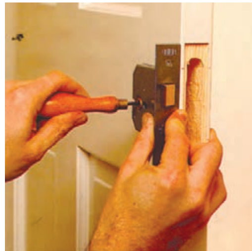
شکل ۱۰-۴۷- علامت‌گذاری پلاک و دستگیره‌ی قفل روی در، با درفش.
