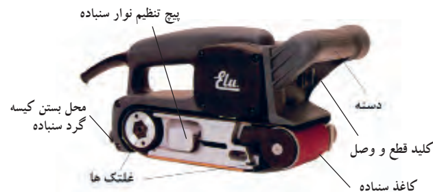
شکل ۷-۵- اجزای مهم و کاربردی دستگاه سنباده نواری.
