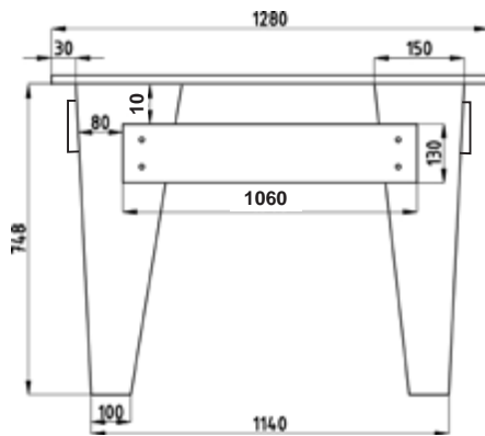
شکل ۱۲-۱۰ نمای (روبرو میز ناها) فوری.
