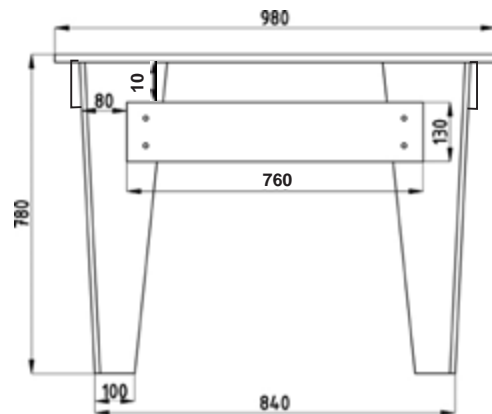
شکل ۱۲-۱۱- نمای جانبی میز ناها (فوری).
