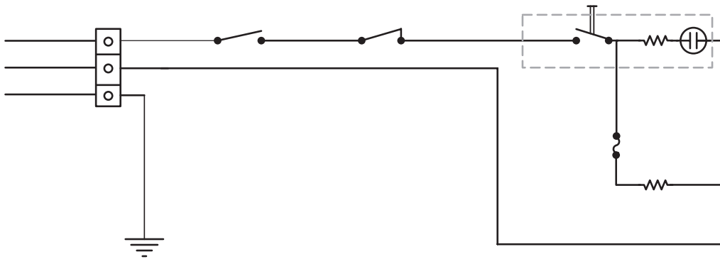
مدار الکتریکی سرخ کن با دیگ چدنی قابل انتقال و شست و شو
