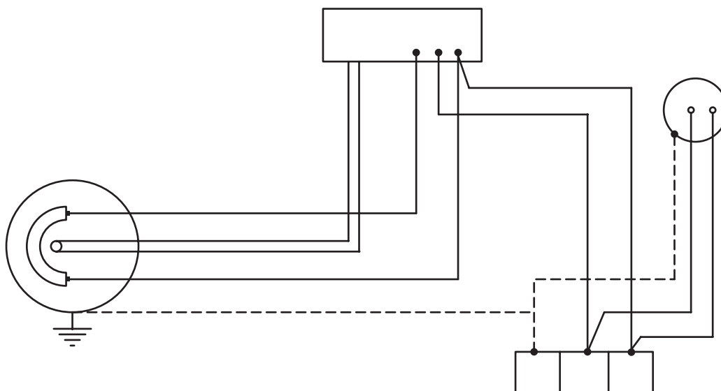
شکل ۱-۷۲ نقشه ی موتناژ چای ساز با صفحه ی نمایشگر
