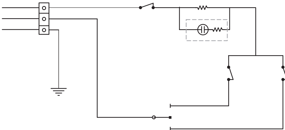
مدار الکتریکی سرخ کن با دو حرارت مختلف ثابت
