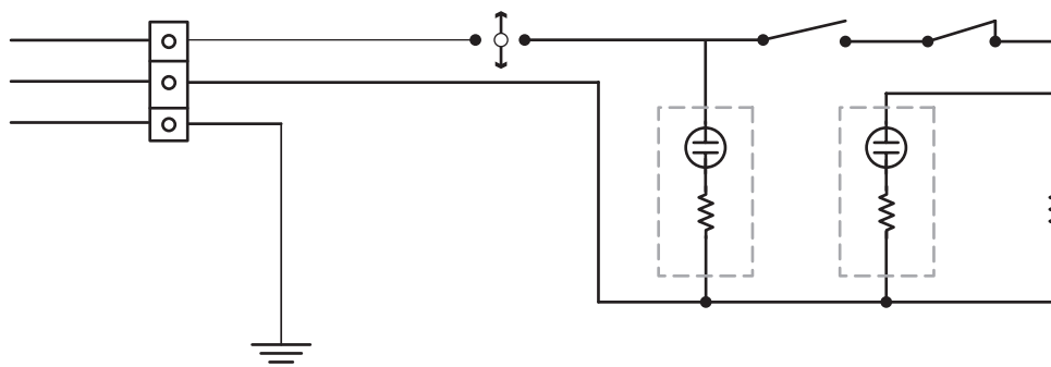
مدار الکتریکی سرخ کن با المنت قابل جدا شدن
