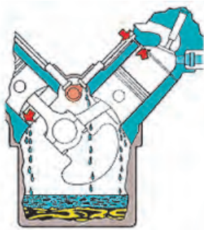
شکل ۲-۹۲- نشتی از اورینگ‌های آب‌بندی پایین بوش سیلندر تر
