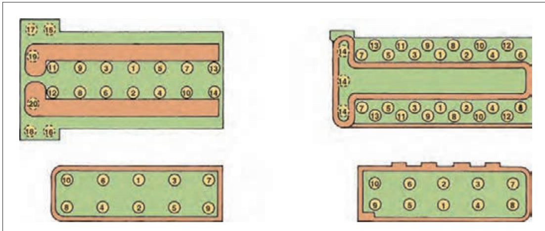
شکل ۳۷-۱. نمونه ترتیب بستن پیچ‌های سرسیلندر
