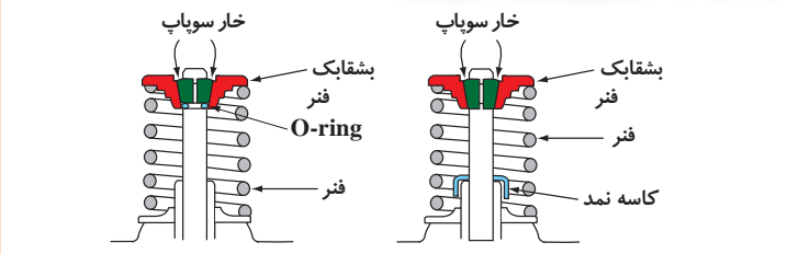
شکل ۱-۷۹- استفاده از اورینگ در گاید
