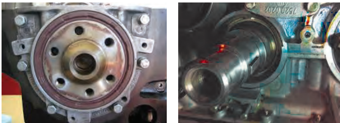
شکل ۴-۱۳- اورینگ و کاسه نمد
