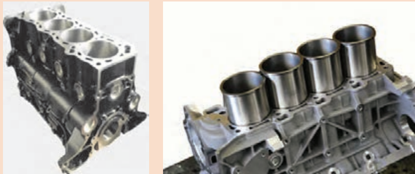
شکل ۲-۲۴- بلوکه با سیلندر یکپارچه و بوش جدا شدنی
