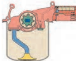
شکل ۱۴۳-۲- پمپ روغن
