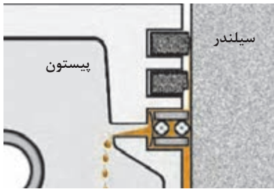
شکل ۲-۴۲- کارکرد رینگ روغنی
