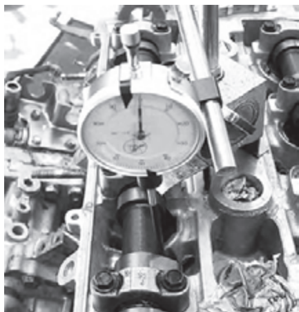
شکل ۱-۷۷- اندازه‌گیری ارتفاع خیز سوپاپ
