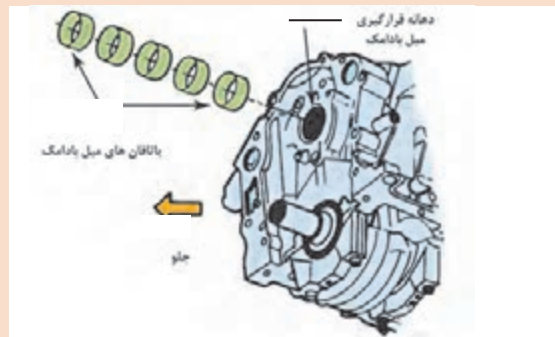
شکل ۷۵-۱- بررسی لقی در یاتاقان یکپارچه
