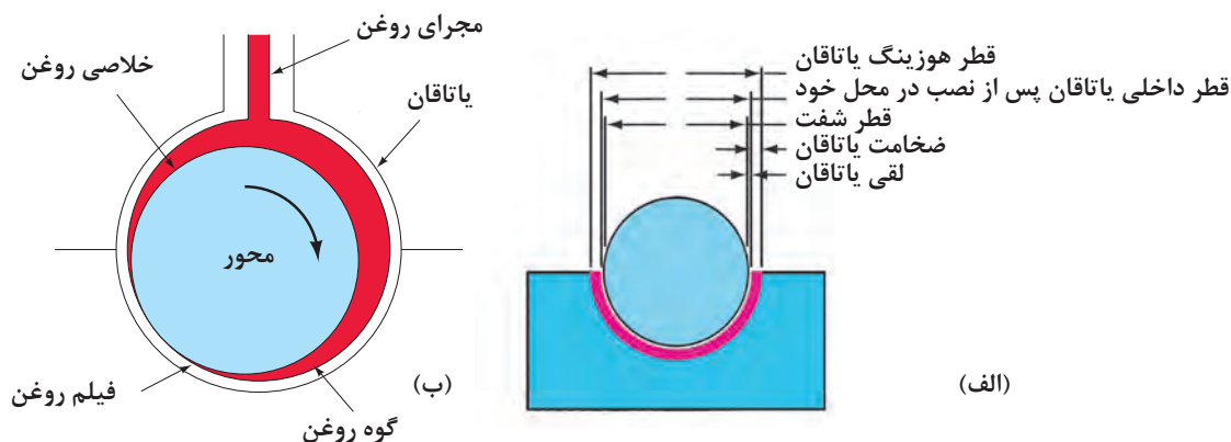
شکل ۸۱-۲- خلاصی بین یاتاقان و میل لنگ (فیلم روغن) در یک یاتاقان
