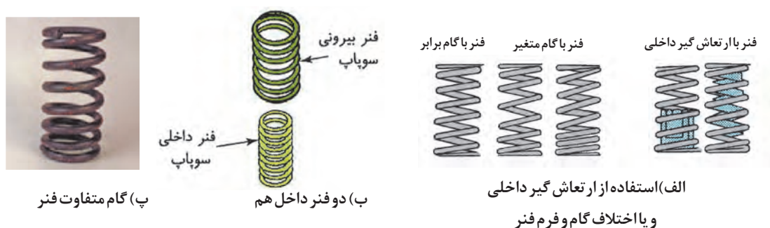
شکل ۸۲-۱- انواع فنر سوپاپ
