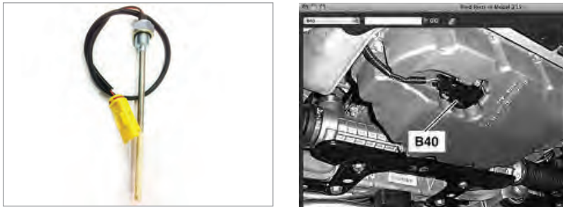
شکل ۱۰-۴- حسگرهای سطح و دمای روغن موتور
