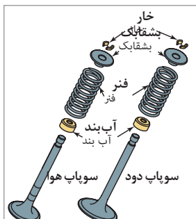
شکل ۱-۸۰- اجزا سوپاپها
