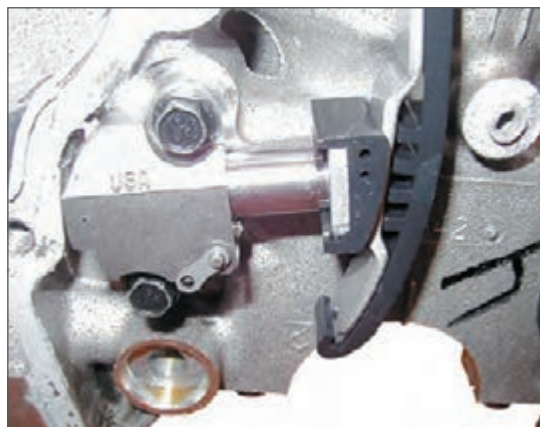
الف) تجهیزات زنجیر سفت کن هیدرولیکی
