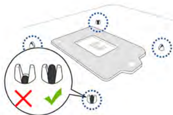
شکل ۳۸- پایه‌های سیستم خنک‌کننده در پشت برد اصلی
