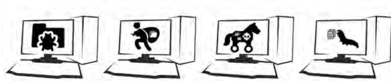
شکل ۲۴- بدافزارها
