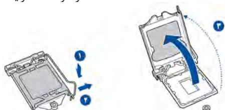
شکل ۳۲- آزاد کردن نگهدارنده سوکت
