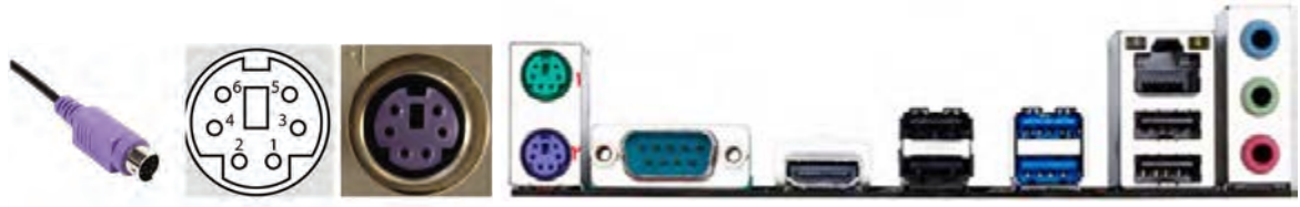
شکل ۸- درگاه‌های روی برد اصلی
